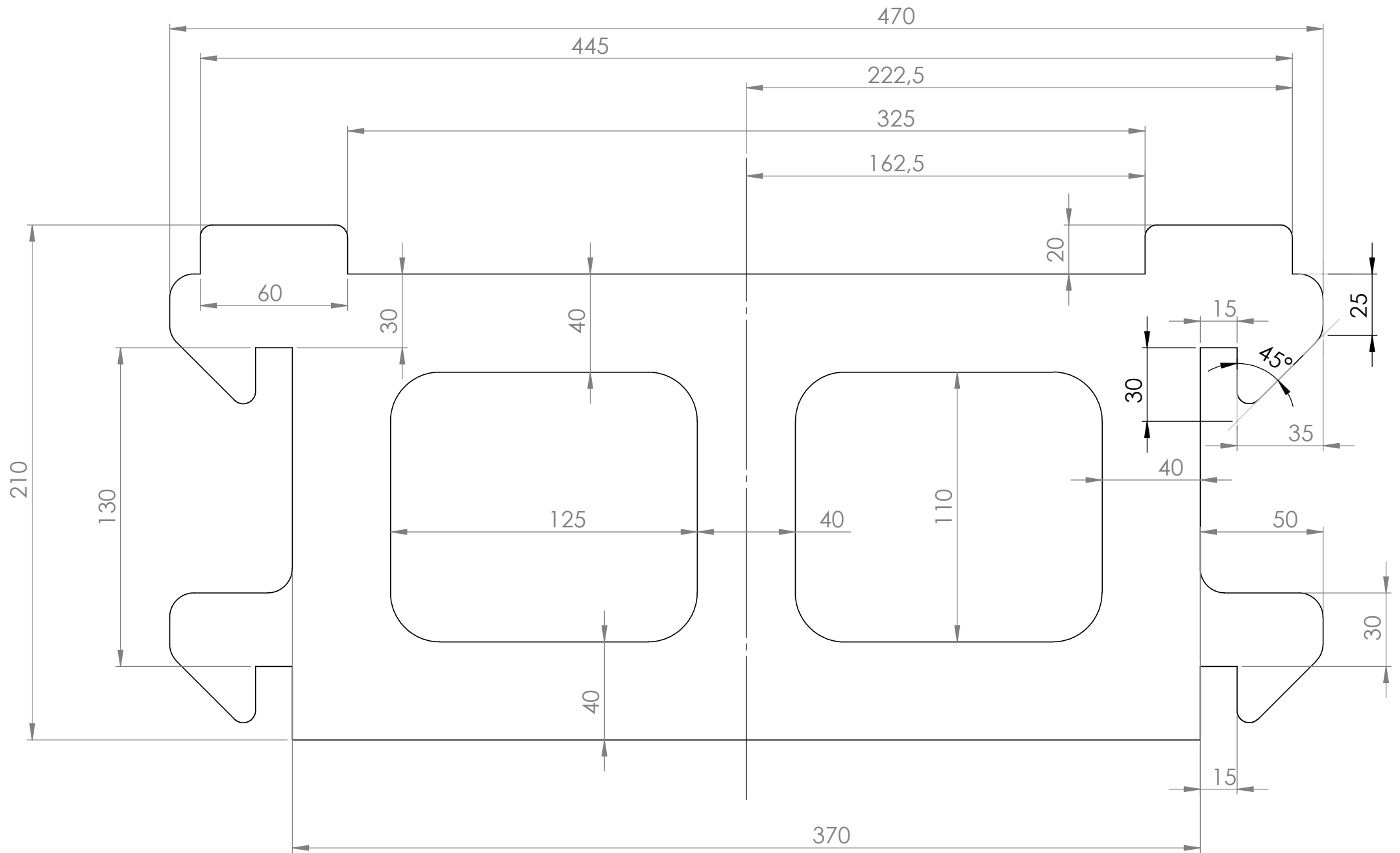
PIECE 3 : TRAVERSE INTERMEDIAIRE
